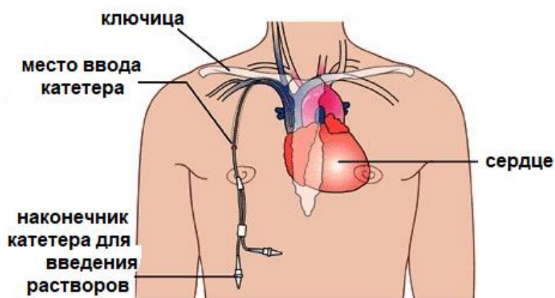
Рисунок 1. Катетер Грошонга.
